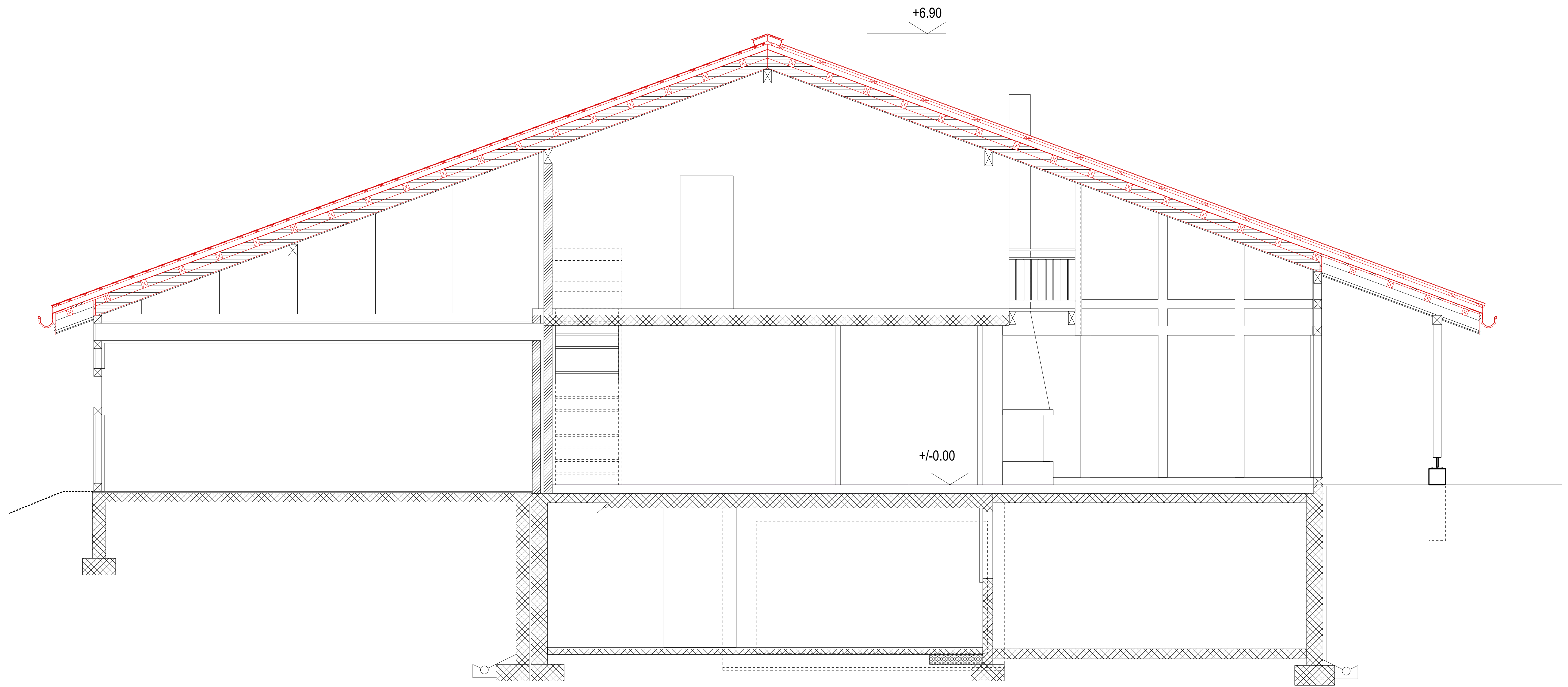
Querschnitt neu 1:33
