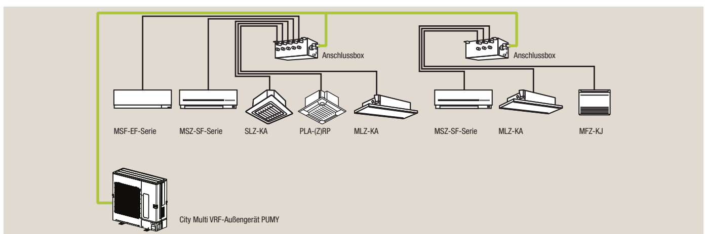
Multisplit-Betrieb mit bis zu 8 Innengeräten aus der M-Serie.
