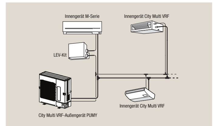
LEV-Kit-Anschluss an City Multi VRF
