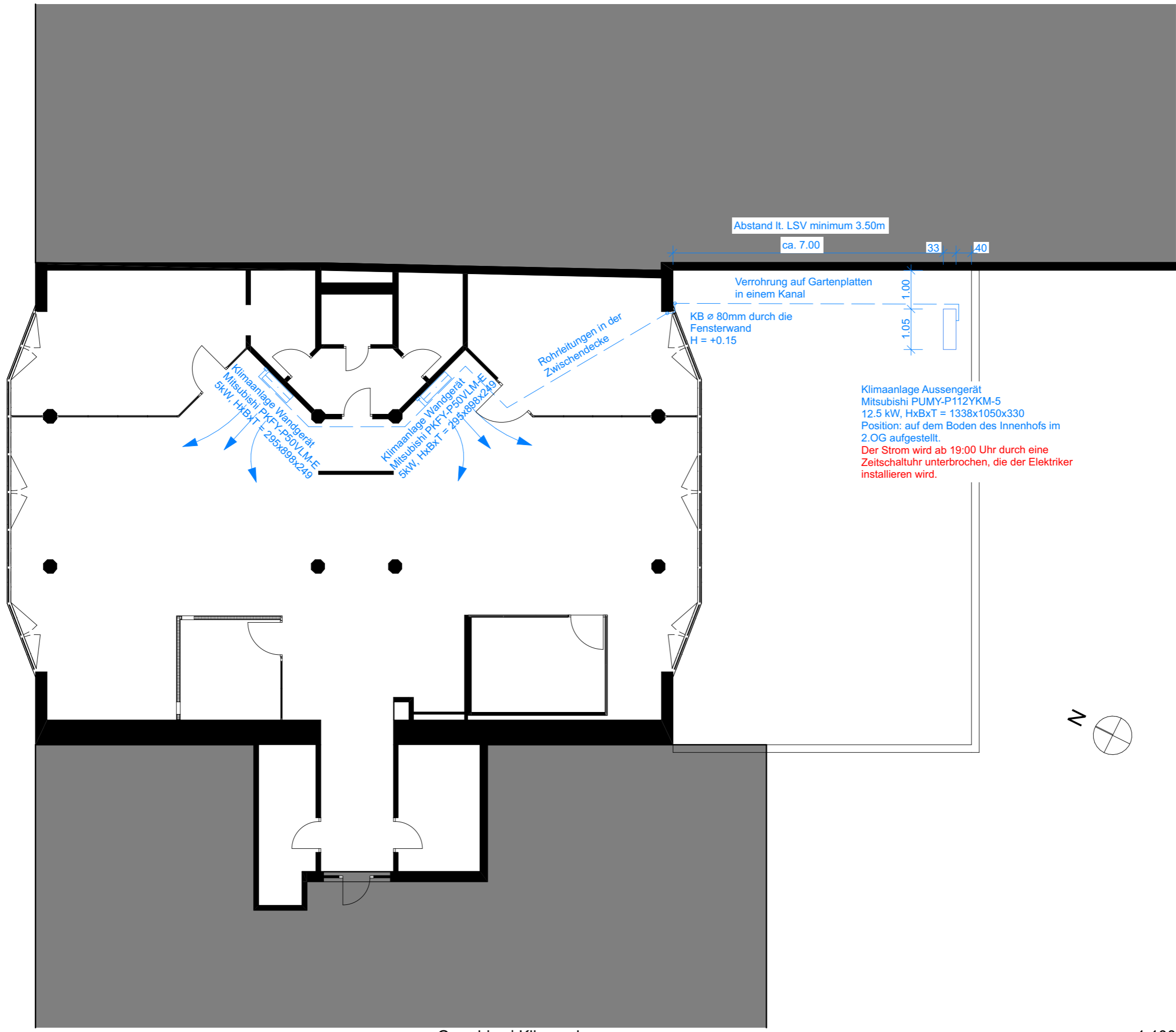
Grundriss | Klimaanlage
