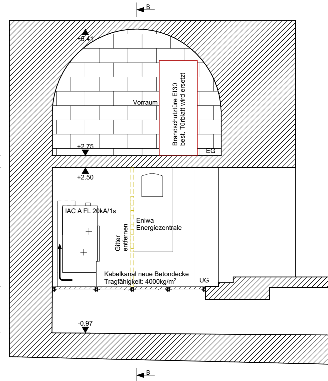
Schnitt A
