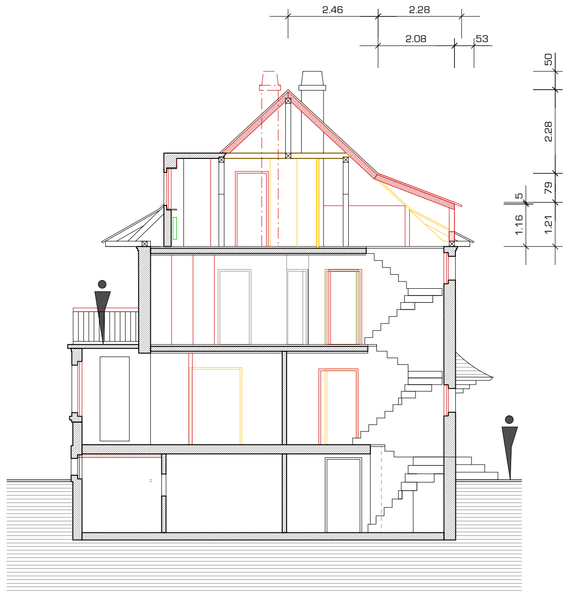
SCHNITT AA / 308.206.01
