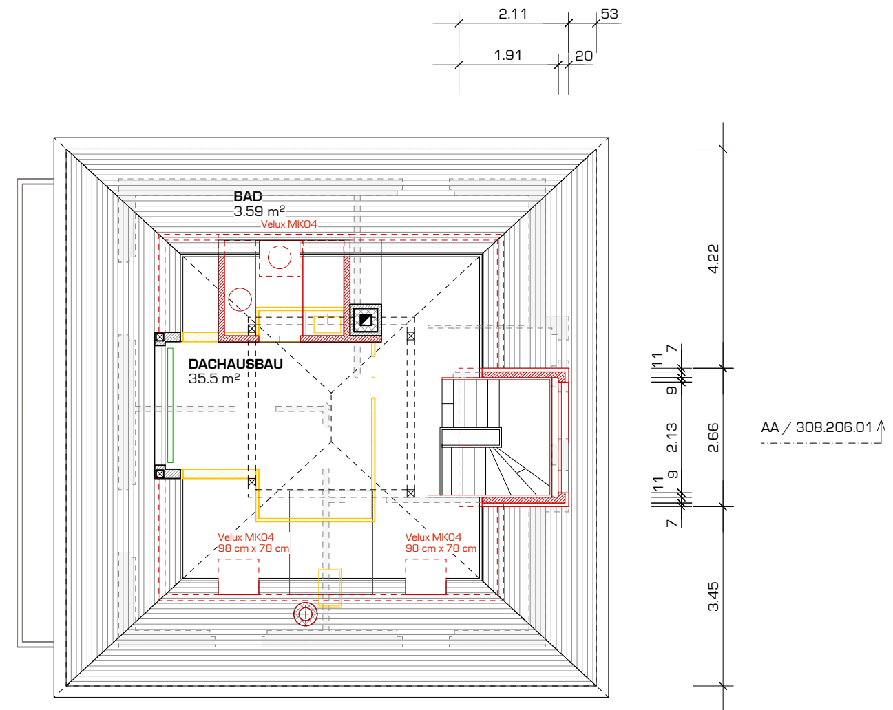
GRUNDRISS DG / 308.202.02
